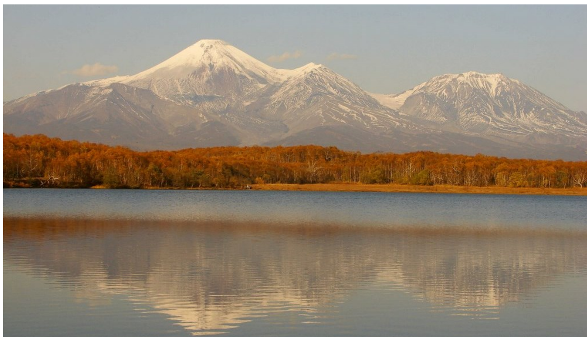
Рис.1 Авачинско-Корякская группа вулканов
